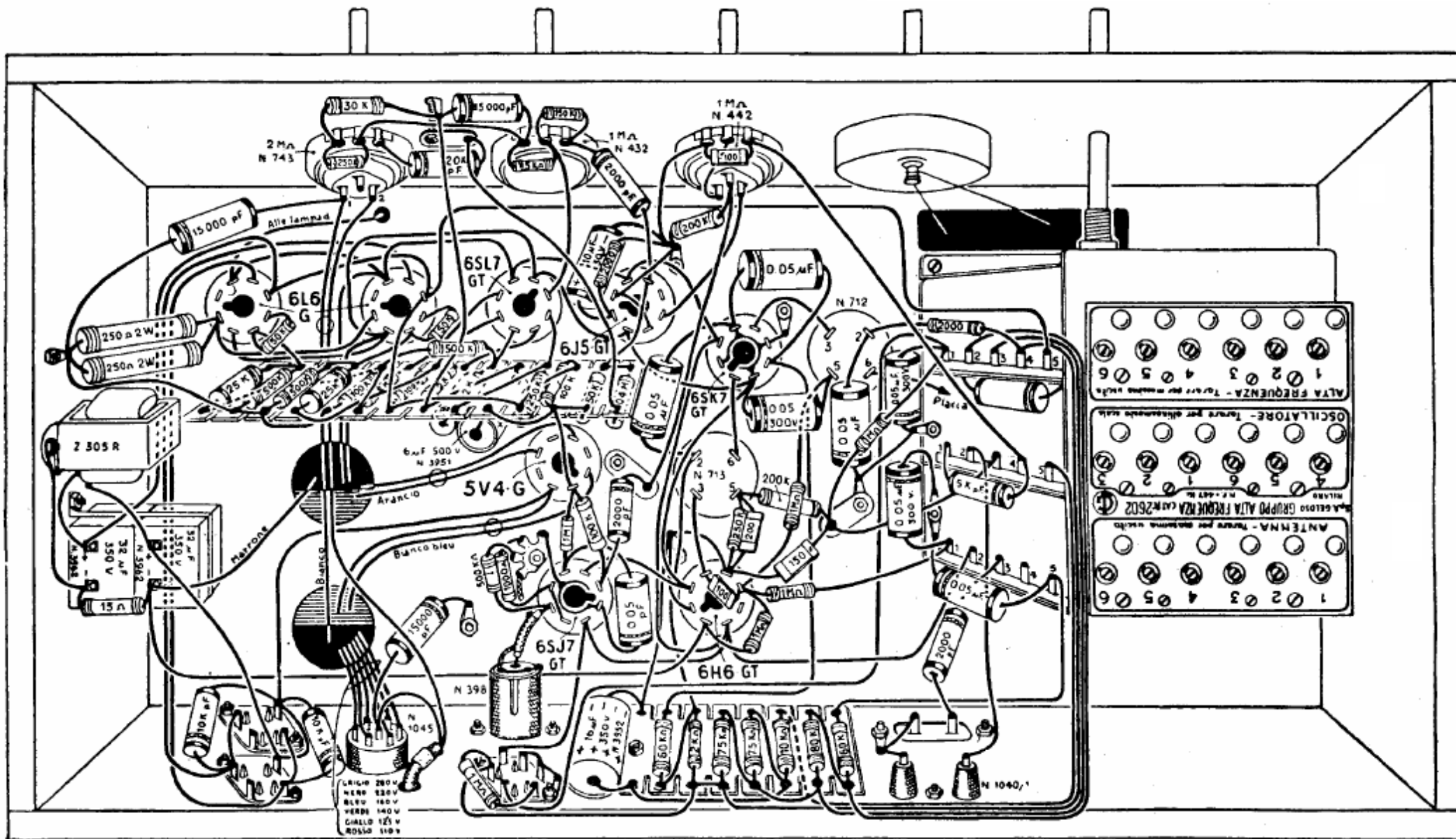
GELOSO - Super G 902 - Piano di montaggio delle parti componenti sottostanti il telaio.
